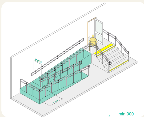
Приклад облаштування входу з пандусом або підймальною платформою (розміри вказані у мм)
