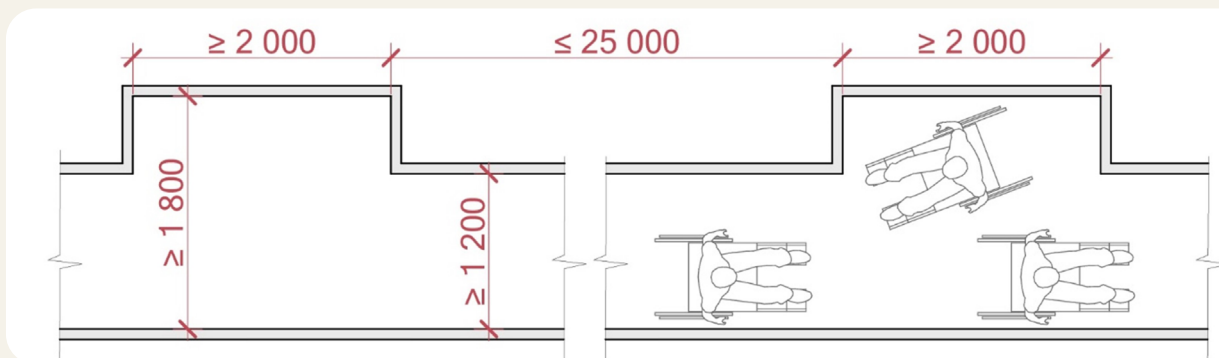
Приклад облаштування пішохідної доріжки з облаштуванням роз'їзних карманів (розміри вказані у мм)
