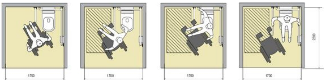
БІЧНЕ ПЕРЕМІЩЕННЯ З РОЗТАШУВАННЯ КІСЛА КОЛІСНОГО ПІД КУТОМ ДО СТІН (З ПРАВОЇ АБО ЛІВОЇ РУКИ). ВАРІАНТ 2
