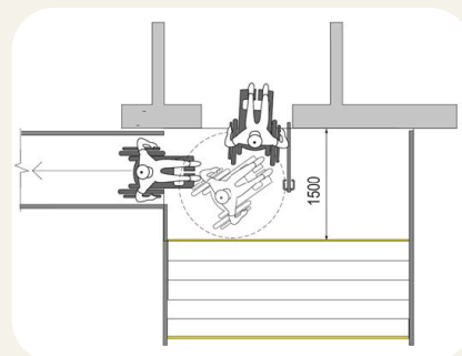
Рисунок 1.22. Схема маневрування кріслом колісним на ганку
