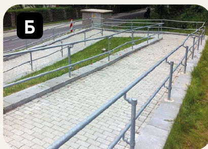
Рисунок 1.18. Приклади покриття пандуса:
