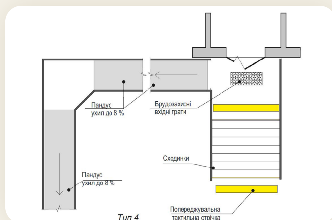
Рисунок 1.23.3. Типи облаштування вхідної групи (продовження): д) П-подібний пандус
