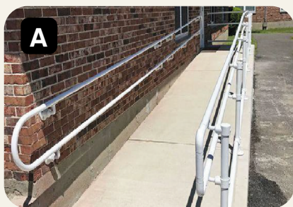
Рисунок 1.18. Приклади покриття пандуса:
