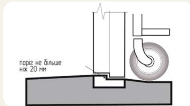
Рисунок 1.9. Поріг вхідного вузла
