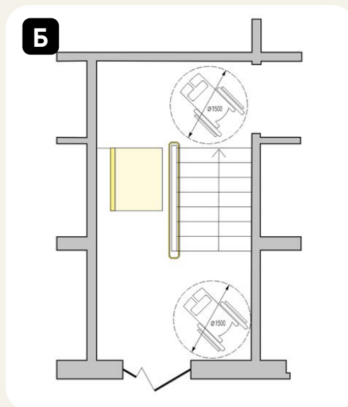
Рисунок 1.40. Схема встановлення підймального пристрою:
