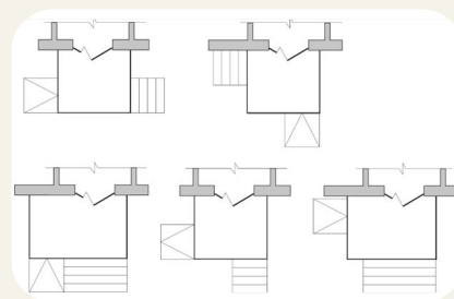
Рисунок 1.20. Рекомендовані схеми взаємного розміщення пандуса і сходів
