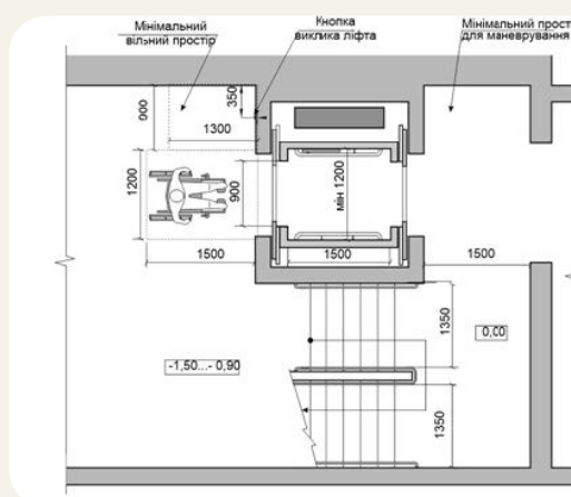
Рисунок 1.45. Ліфт з прохідною кабіною
