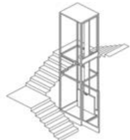
Приставний ліфт
