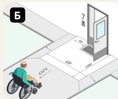
Рисунок 1.4. Приклади забезпечення входу в будинок з рівня вимощення Вхідні двері
