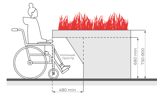
Відповідна конструкція діжки для інвалідного візка
