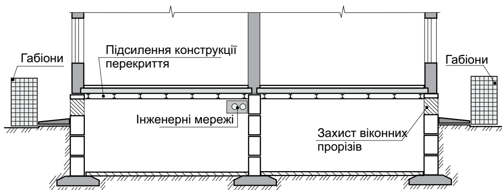
Рис. 22. Укриття в підвальному приміщенні цегляних будинків із залізобетонним перекриттям
