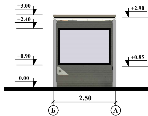
ФАСАД Б-А М 1:75
