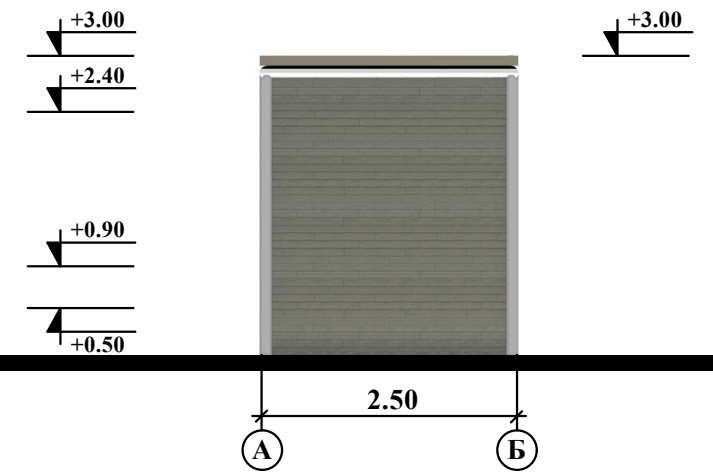
ФАСАД А-Б М 1:75
