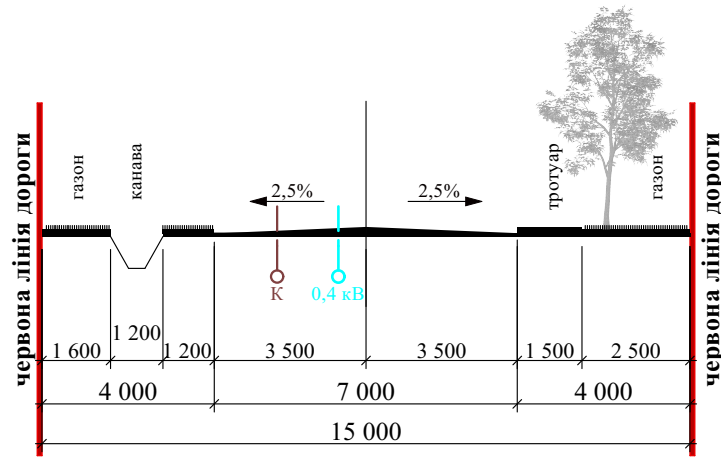
Розріз I-I по вул. Біласа і Данилишина М 1:200
