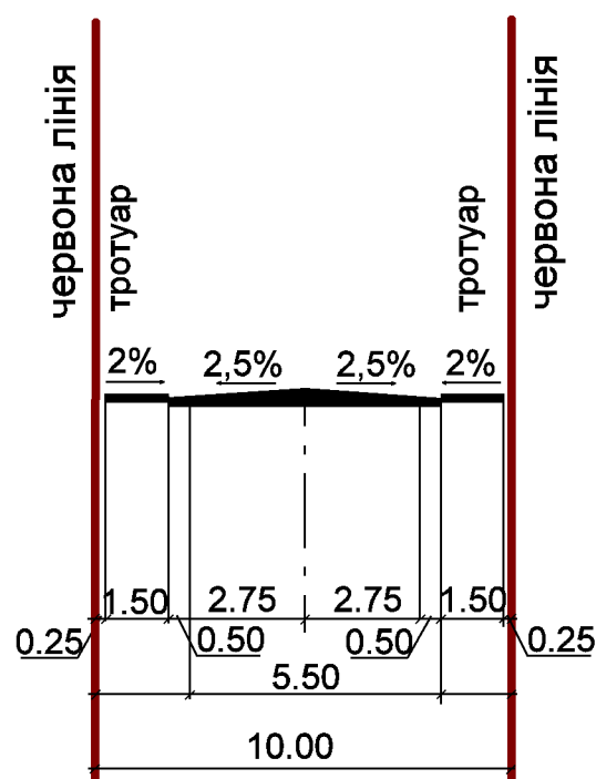
Розріз II-II
