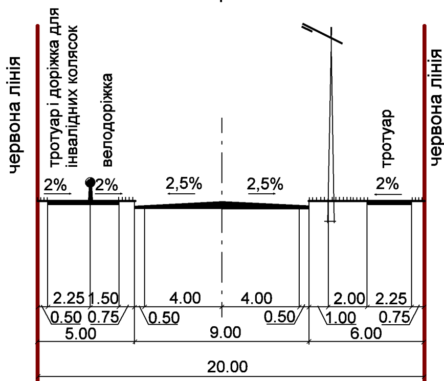
Розріз І-І
