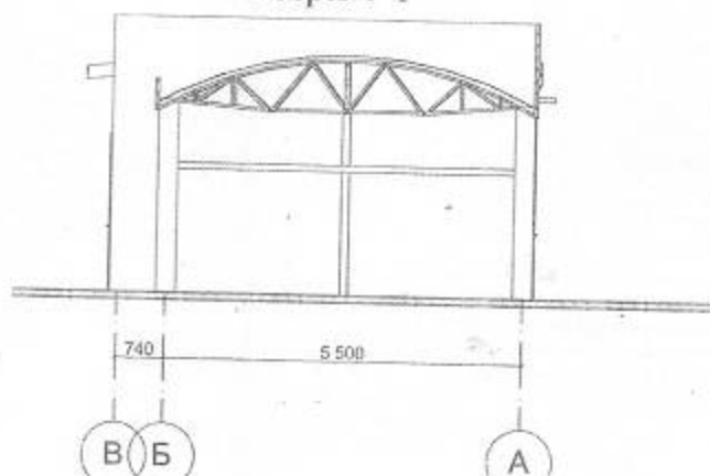
Розріз 1-1
