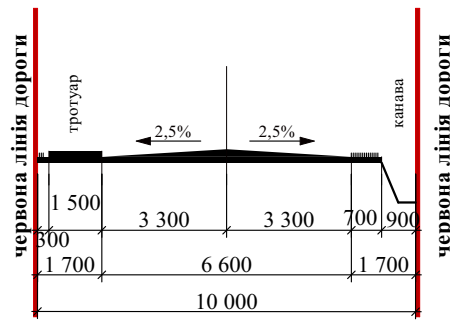
Розріз II-II по вул. Фінська М 1:200
