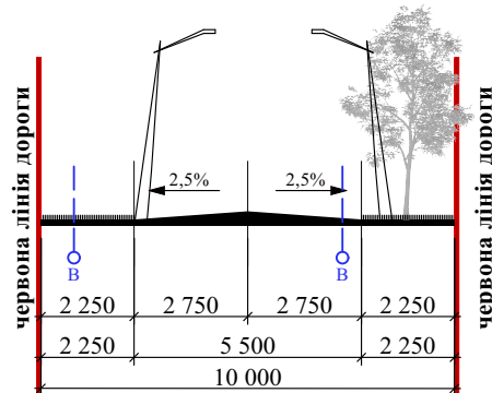
Розріз III-III по вул. Космонавтів М 1:200
