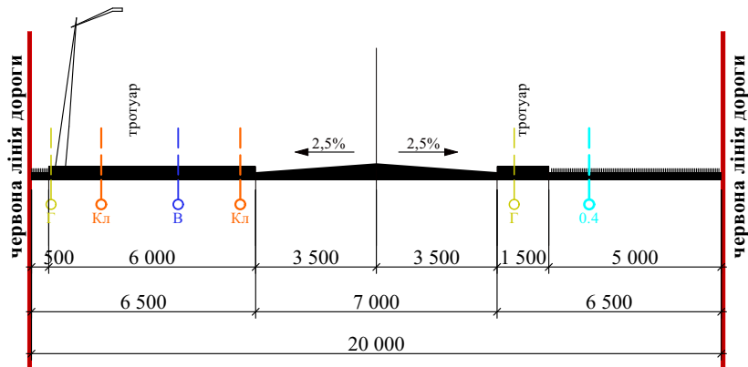
Розріз I-I по вул. Хіміків М 1:200
